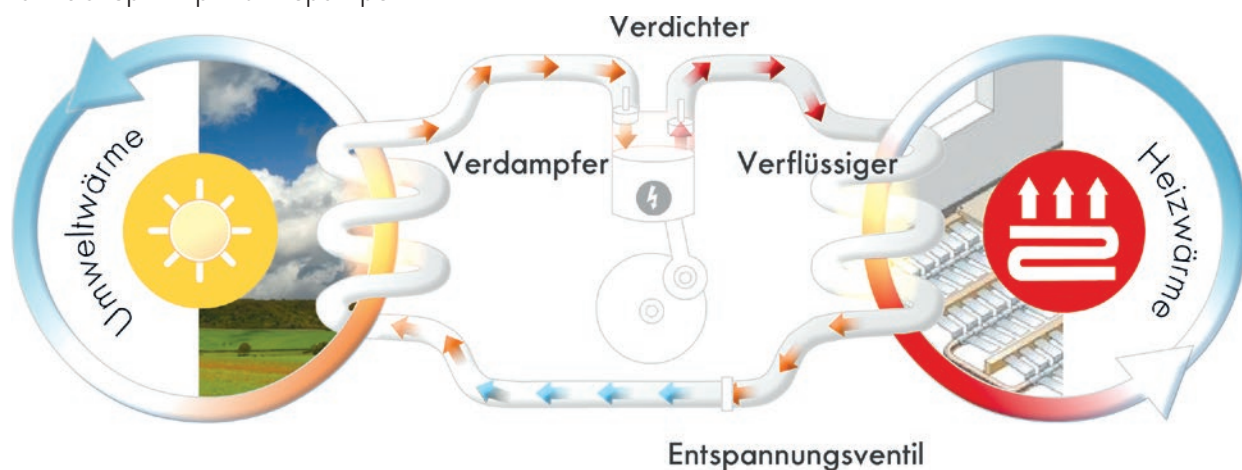
Funktionsprinzip Wärmepumpe
